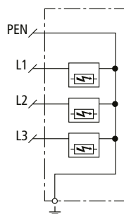
Prinzipschaltbild DSH ZP B2 TNC 255
