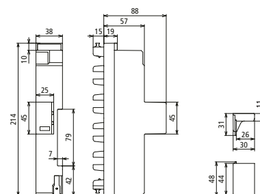
Maßbild DSH ZP B2 TNC 255
