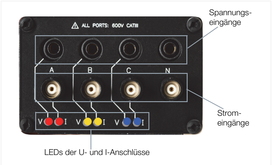
Bild 3: Geräteoberseite
