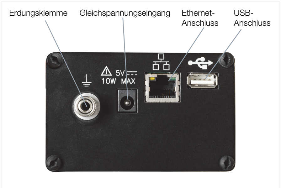
Bild 4: Geräteunterseite
