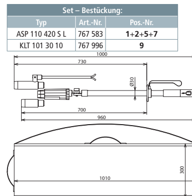
Maßbild ASPS 110 420 S L
