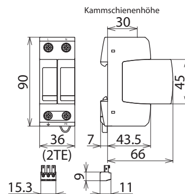
Maßbild DG M TN 275 FM
