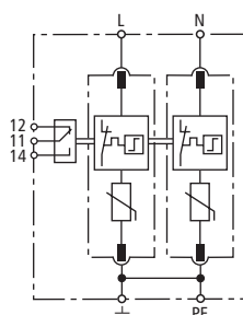
Prinzipialschaltbild DG M TN 275 FM
