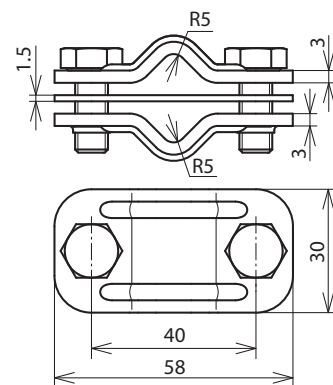
Maßbild ZMTK 8.10 8.10 CU STTZN
