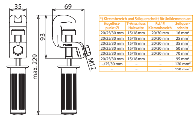
Maßbild UEK 25 HG
