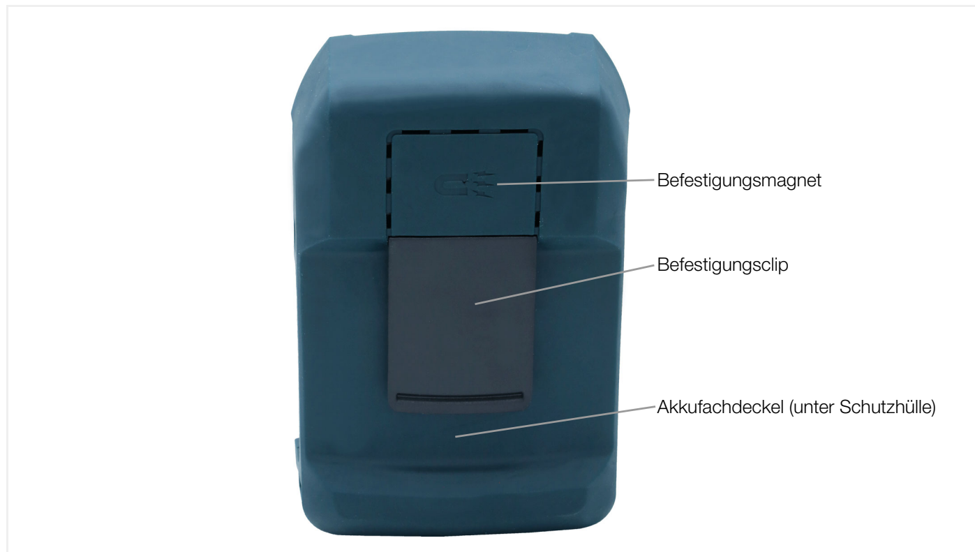
Bild 4: Geräterückseite
