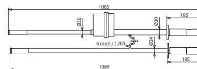
Maßbild PHEG2 P SN7194
