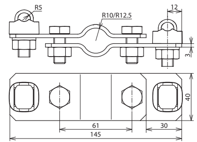
Maßbild AS TE 20 2XKSV 7.10 STTZN
