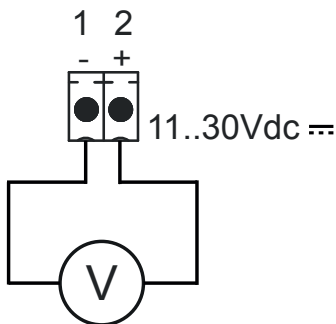
Anschlussschema BT7050
