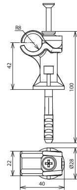
Maßbild SH DFI 16 STTZN H42 GR
