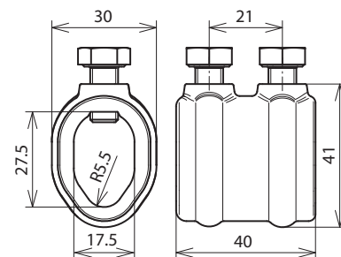
Maßbild TM 7.10 16 ZG
