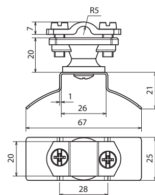
Maßbild LH ZS 6.11 SBB PA V2A
