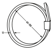
Maßzeichnung perspektivisch
