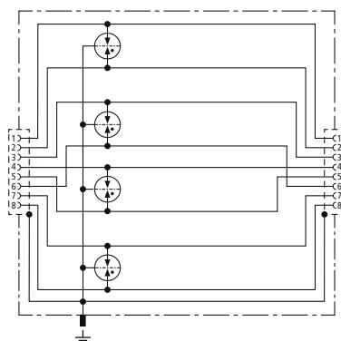
Prinzipschaltbild DPA C8 D 4PPOE
