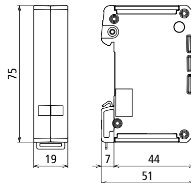
Maßbild DPA C8 D 4PPOE
