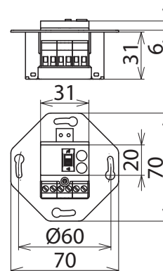
Maßbild DSA 230 LA
