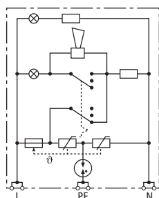
Prinzipschaltbild DSA 230 LA
