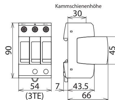
Maßbild DG M YPV SCI 1000
