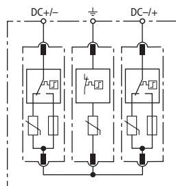
Prinzipialschaltbild DG M YPV SCI 1000
