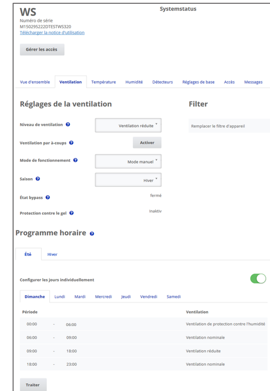
Fig. Réglages de la ventilation jusqu'à la version du micrologiciel 1.2.7
