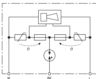
Prinzip Schaltbild DFL M 255
