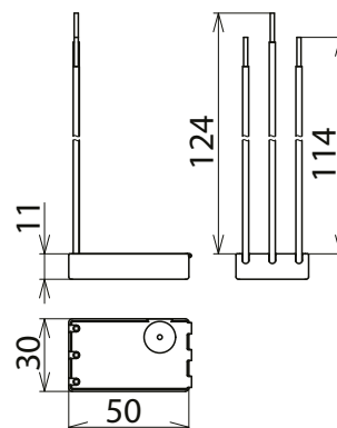
Maßbild DFL M 255
