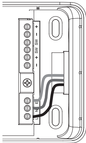
Vorderansicht: Unterputz Verdrahtung
