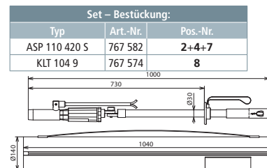
Maßbild ASPS 110 420 S
