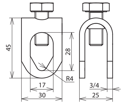
Maßbild FSK 8.10 16 SKM10X25 STTZN
