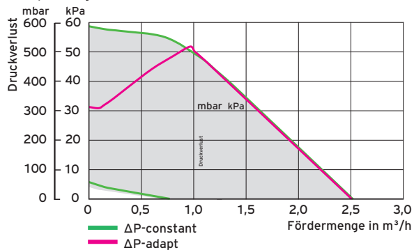
Pumpendiagramm Einbau-Sets eco/auroCOMPACT
