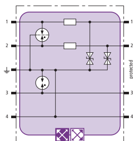
Prinzipschaltbild BXT ML2 BE S 24
