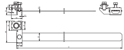
Maßbild BRS 27.168 Z AK1X10 2X6.8 V2A
