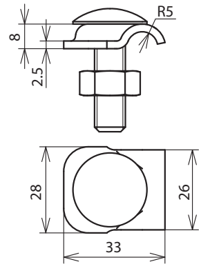
Maßbild KB 6.10 FRM10X35 V2A
