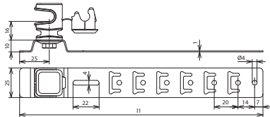
Maßbild DLH US 8 H16 L335 GR V2A
