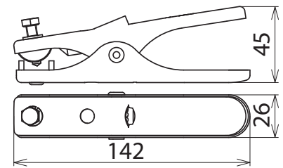
Maßbild
