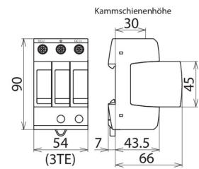
Maßbild DG M YPV SCI 150
