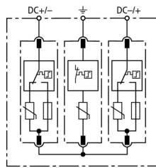
Prinzipialschaltbild DG M YPV SCI 150
