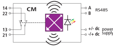
Prinzipialschaltbild DRC MCM AL XT
