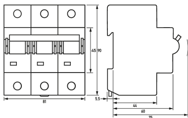
Maßzeichnung Gruppenansicht
