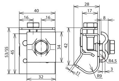
Maßbild DRK DUL 8.10 W16.22 AL
