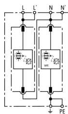
Prinzip Schaltbild DV M TT 2P 255
