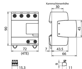
Maßbild DVA EMOB M 3P 255 FM
