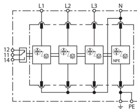
Prinzipialschaltbild DVA EMOB M 3P 255 FM
