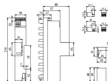
Maßbild DSH ZP B2 SG TNS 255
