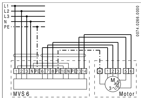
Bilde 2: Koplingsskjema
