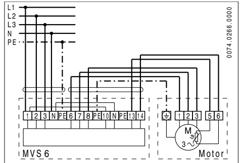
Bild 2: Anschluss-Schaltbild
