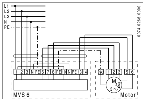
Εικόνα 2: Διάγραμμα σύνδεσης
