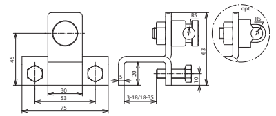
Maßbild AK 6.10 KSV S KBF3 18 V2A
