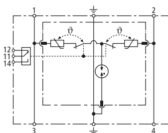
Prinzipschaltbild DR M 2P 255 FM
