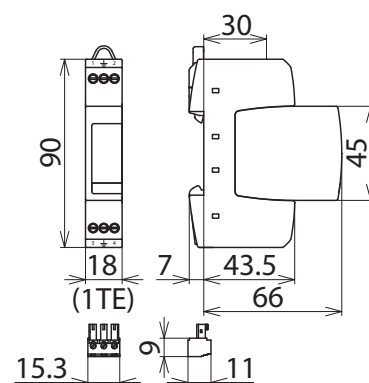
Maßbild DR M 2P 255 FM
