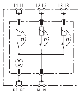
Prinzipschaltbild DR M 4P 255
