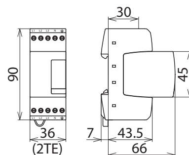
Maßbild DR M 4P 255
