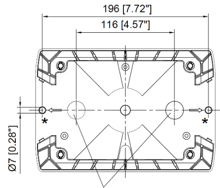
M20-Ausbruch vorbereitet
