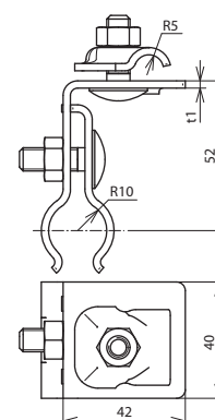
Maßbild DLH KB 6.10 RSF20.25 AL
