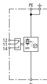
Prinzipschaltbild DGPM 1 255 FM
