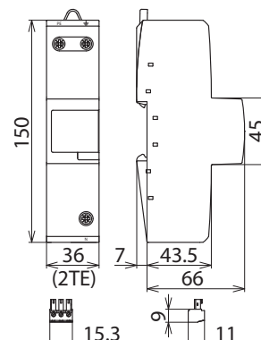
Maßbild DGPM 1 255 FM
