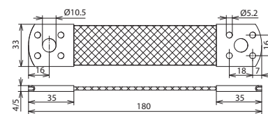
Maßbild UEBB L180 B10.5 B5.2 AL
