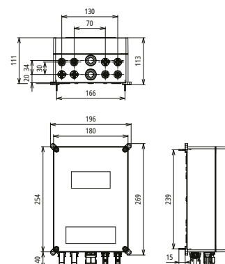
Maßbild DCU 2 YPV 1+2 1200 2M 1S MC4
