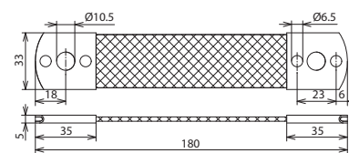
Maßbild UEBB L180 B10.5 B6.5 AL
