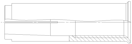
Dübelhülse
