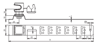
Maßbild DLH US 8 H16 L205 GR V2A
