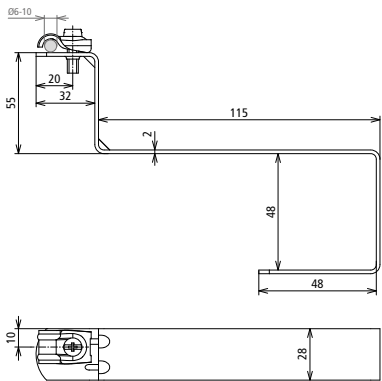
Maßbild DLH DQ 6.10 H55 L115 WS STTZN
