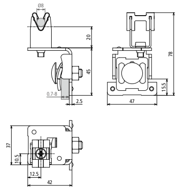
Maßbild DLH DG 8 SF0.7 8 V2A
