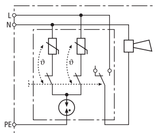
Prinzipschaltbild DFL A 255
